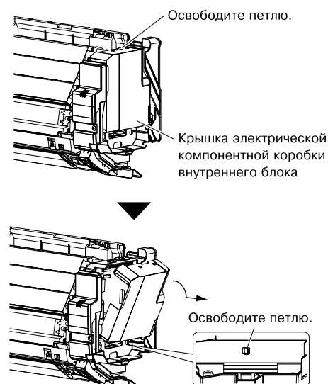
Рисунок 1: Снимите крышку с электрической компонентной коробки внутреннего блока
